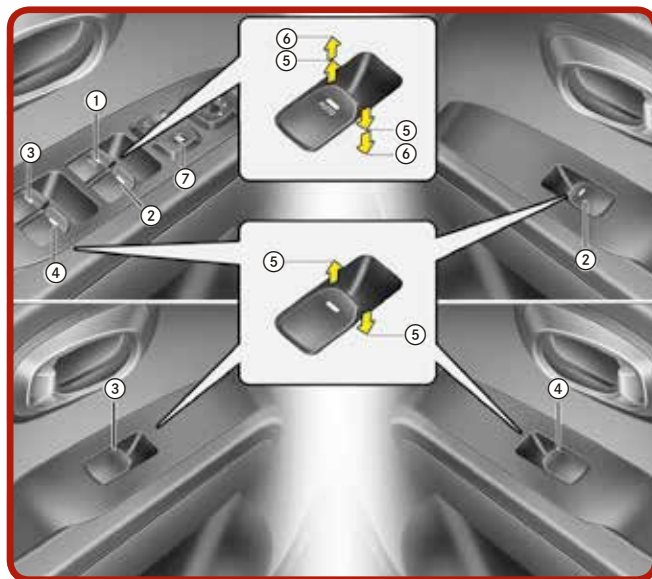
Alzacristalli [4]
