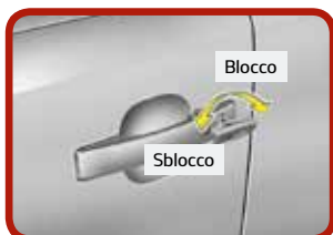
Azionamento manuale delle serrature delle porte [4]
