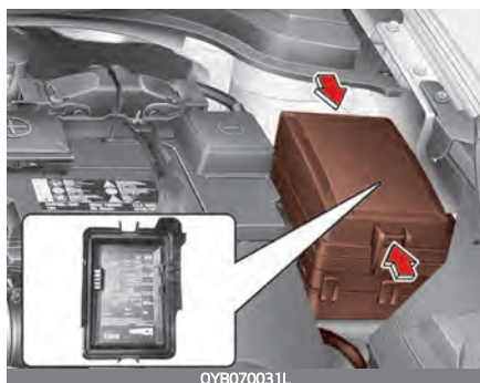
Scatola fusibili vano motore (Smartstream G1.0 T-GDi PTC solo riscaldatore)
