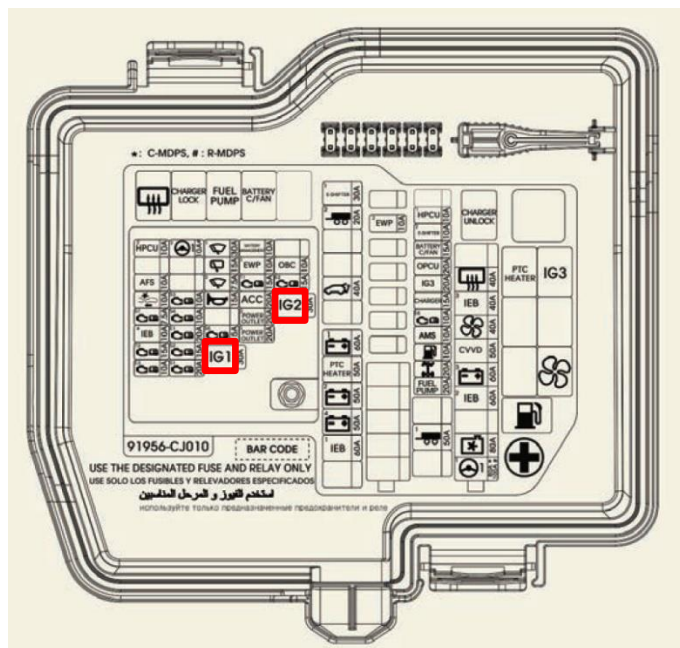
Κιβώτιο ασφαλειών χώρου κινητήρα
