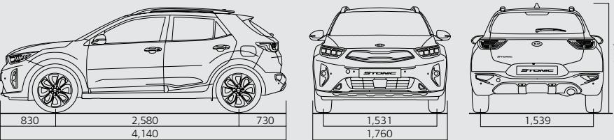
Διαστάσεις (mm)
