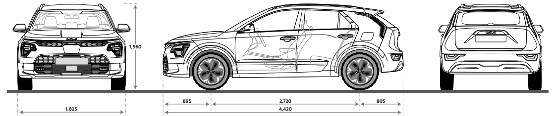
Dimensions Niro EV 100 % électrique (mm)
