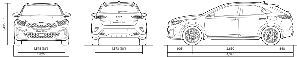
Dimensiones GT-line (mm)
