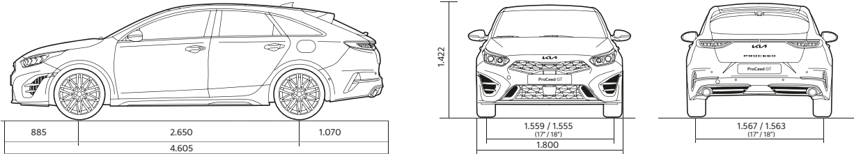
Abmessungen ProCeed (in mm)
